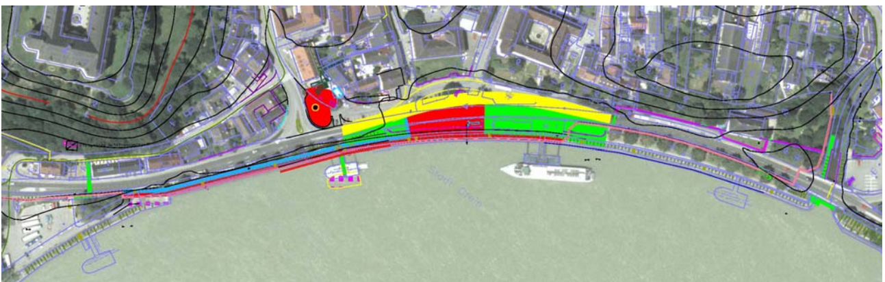
Hochwasserschutz Machland Damm Lageplan Kaigestaltung Grein
